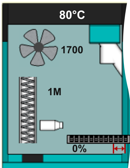
Keine Flamme
