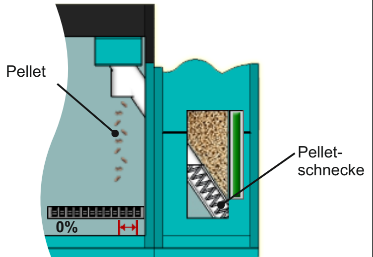
Pelletschnecke arbeitet (Pellets fallen und Schnecke bewegt sich)
